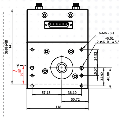
入光板和安装板
