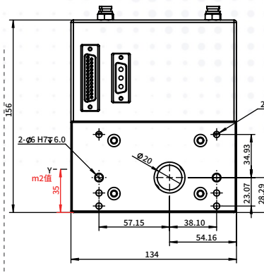
入光板和安装板
