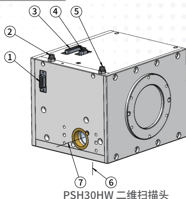
PSH30HW 二维扫描头
