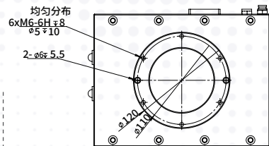
机械臂安装尺寸
