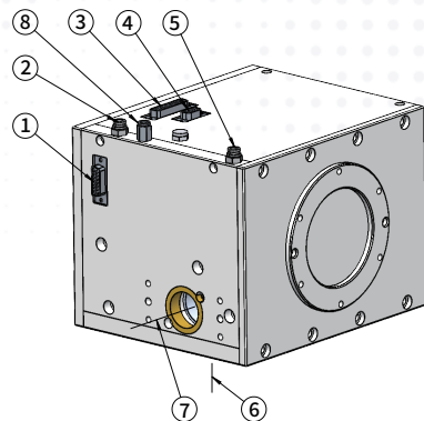
PSH30HWA 二维扫描头
