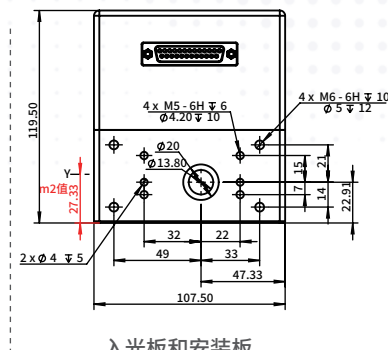
入光板和安装板
